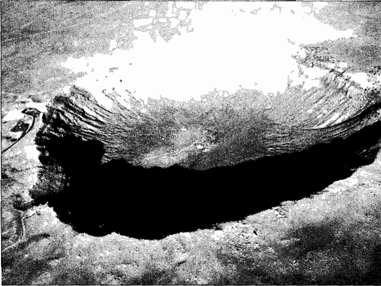
الحفرة التي أحدثها سقوط النيزك كارتر في أريزونا
